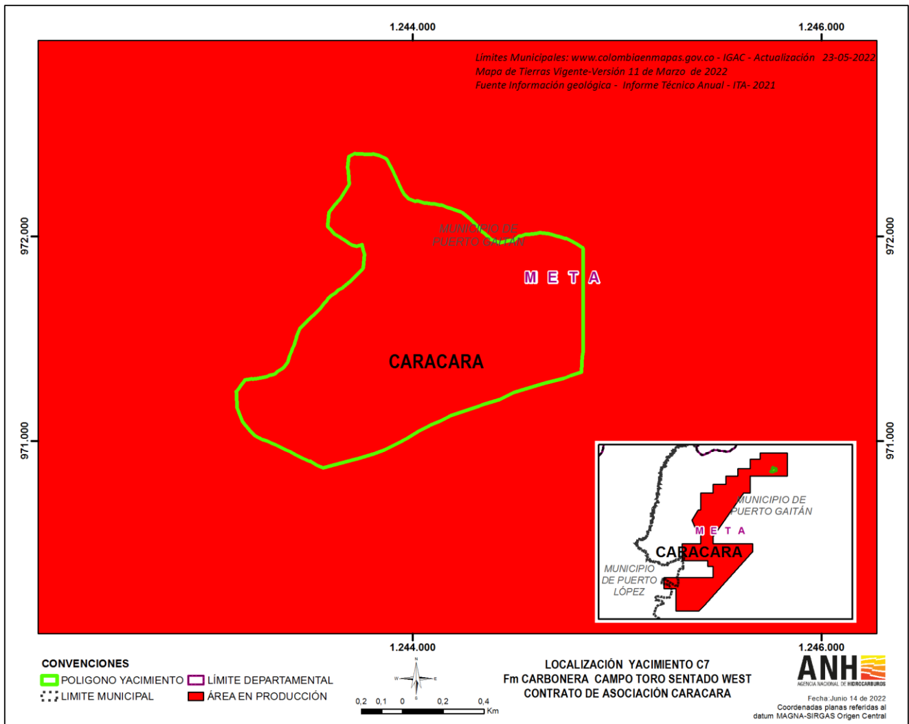
Figura. Localización Yacimiento C7 Fm Carbonera – Campo Toro Sentado West
