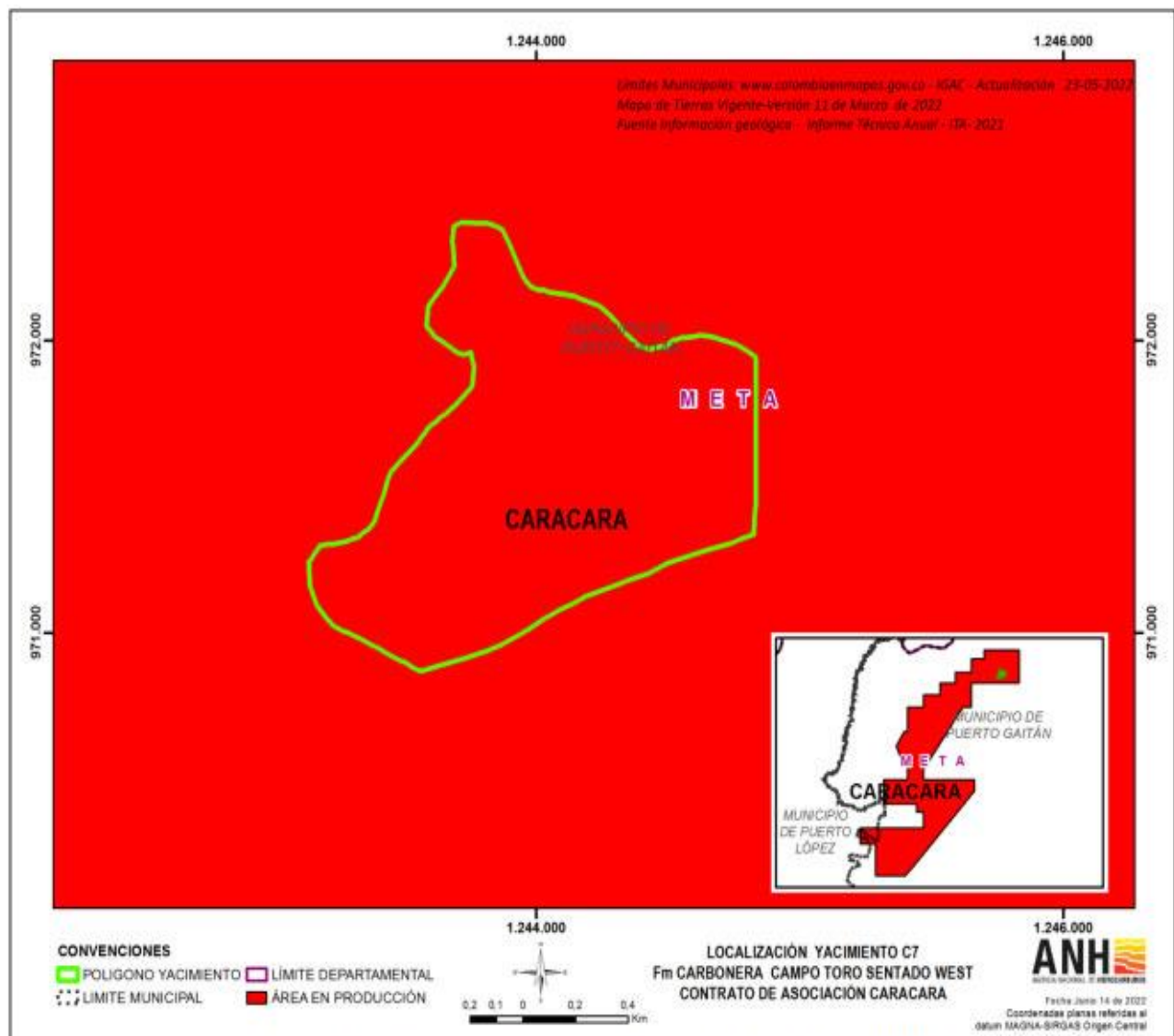
Figura. Localización Yacimiento C7 Fm Carbonera – Campo Toro Sentado West
