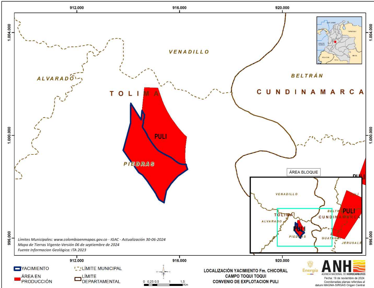
Figura 2. Localización Yacimiento Formación Chicoral – Campo Toqui - Toqui
