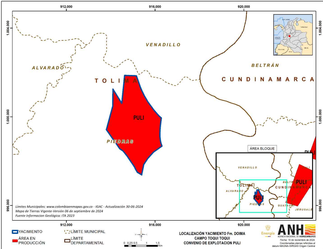
Figura 1. Localización Yacimiento Formación Doima – Campo Toqui - Toqui
