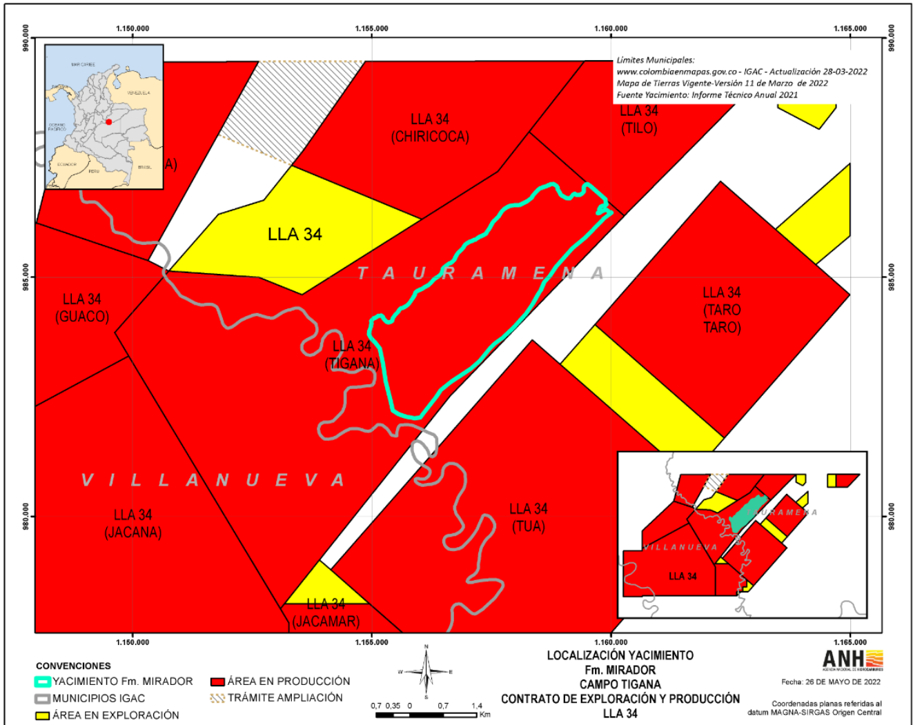
Figura 2. Localización Yacimiento Fm Mirador – Campo Tigana.
