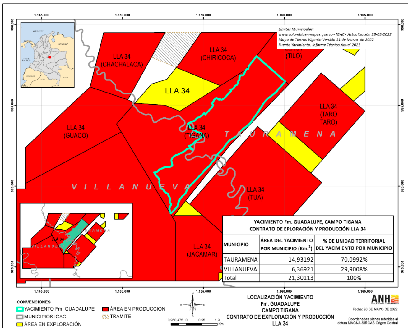
Figura 1. Localización Yacimiento Fm Guadalupe – Campo Tigana.
