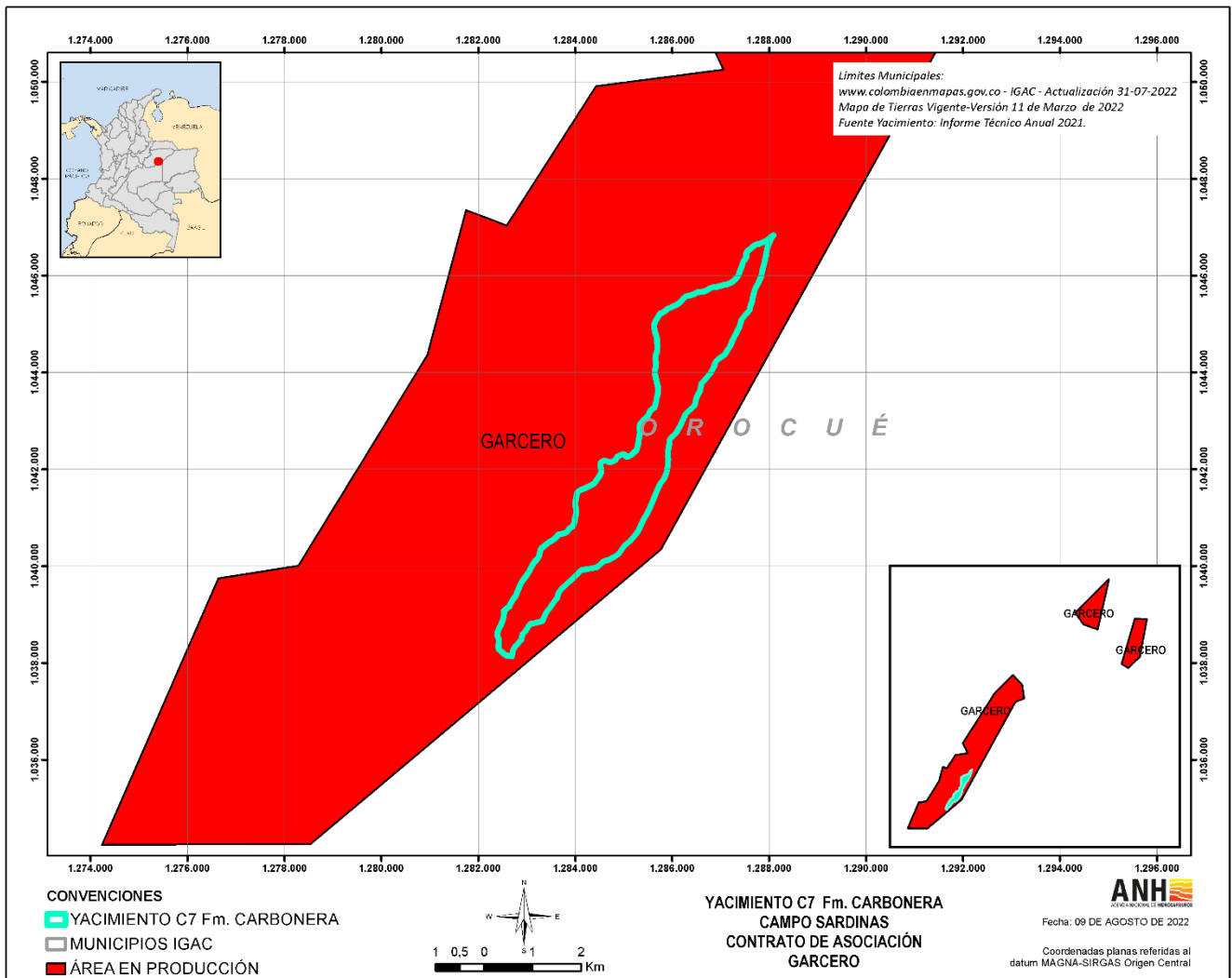
Figura 1. Localización Yacimiento C7 Formación Carbonera – Campo Sardinas.
