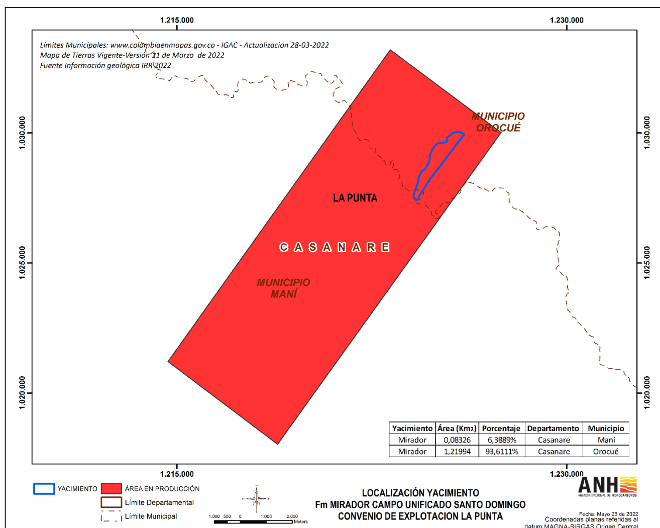
Figura. Localización Yacimiento de la Fm Mirador – Campo Unificado Santo Domingo
