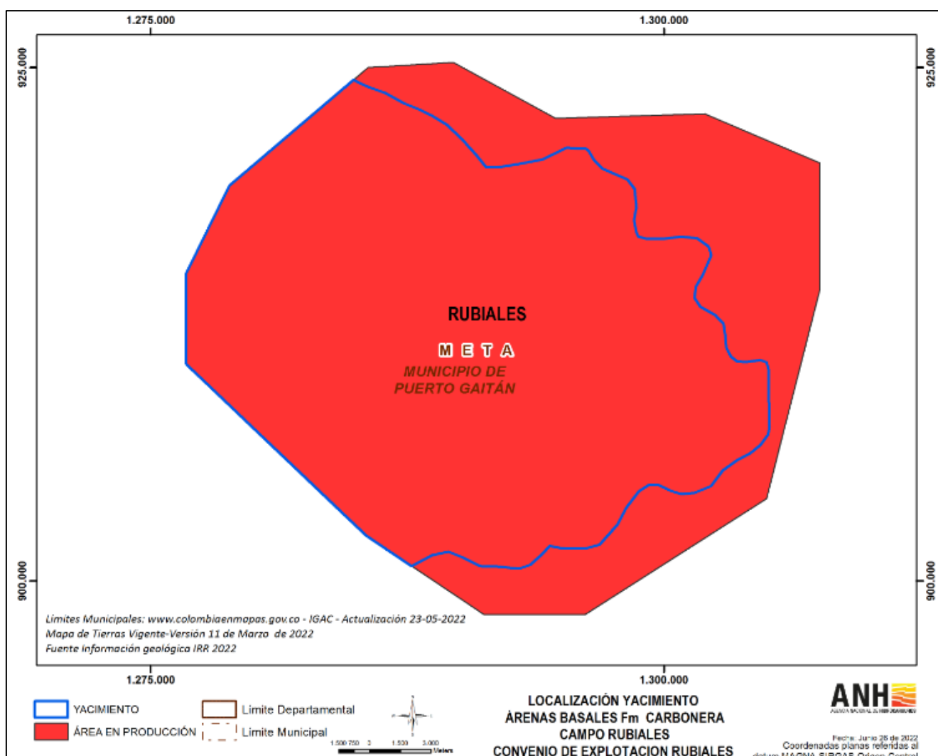
Figura. Localización Yacimiento Arenas Basales. Fm Carbonera – Campo Rubiales
