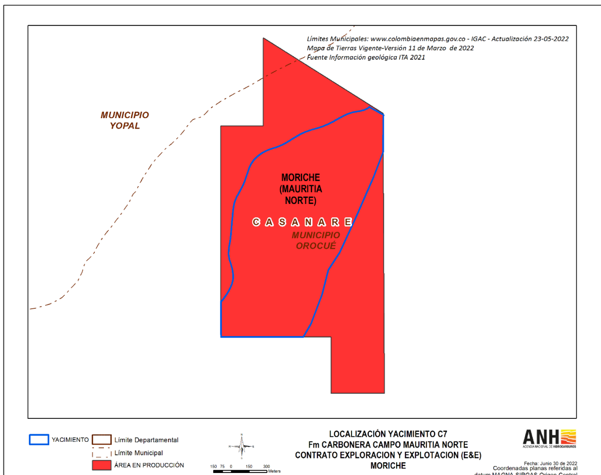
Figura. Localización Yacimiento C7 de la Fm Carbonera C7 – Campo Mauritia Norte
