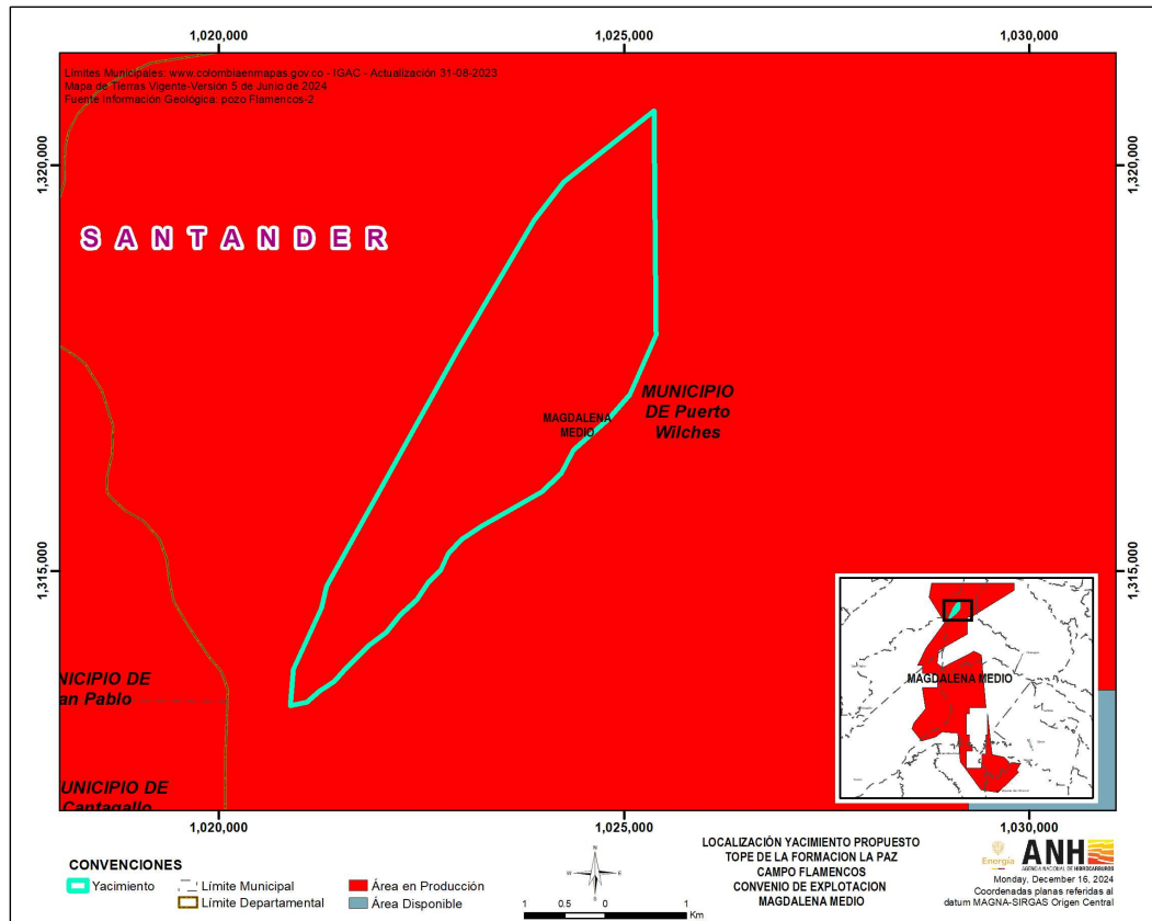
Figura. Localización Yacimiento Arenas Basales de la Formación la Paz – Campo Flamencos”
