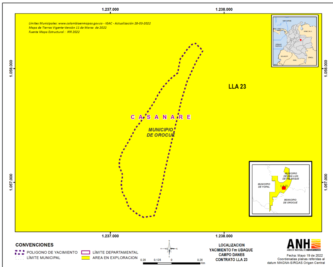
Figura 2. Localización Yacimiento Fm Ubaque – Campo Danés, Contrato LLA 23.
