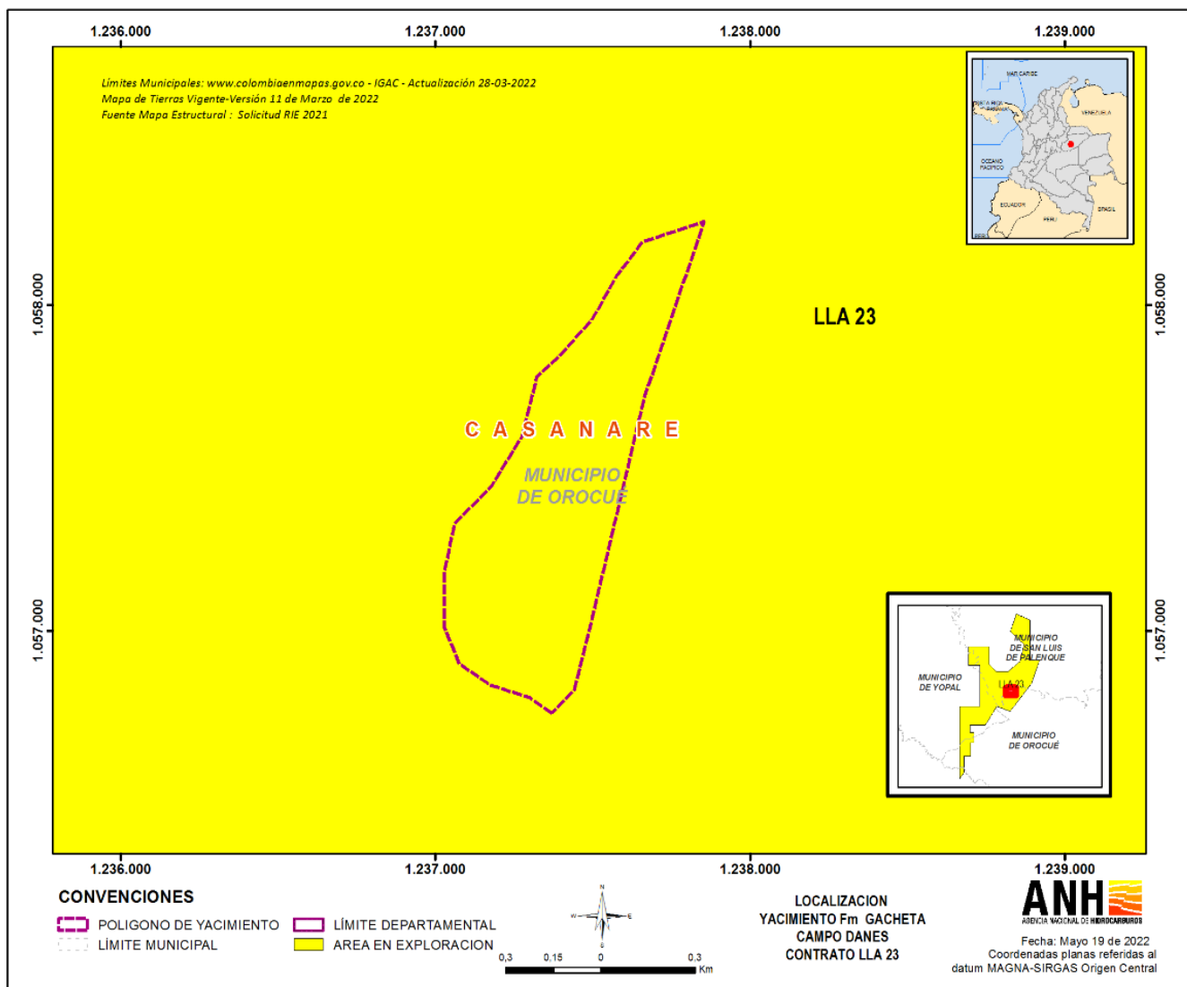
Figura 1. Localización Yacimiento Fm Gachetá – Campo Danés.
