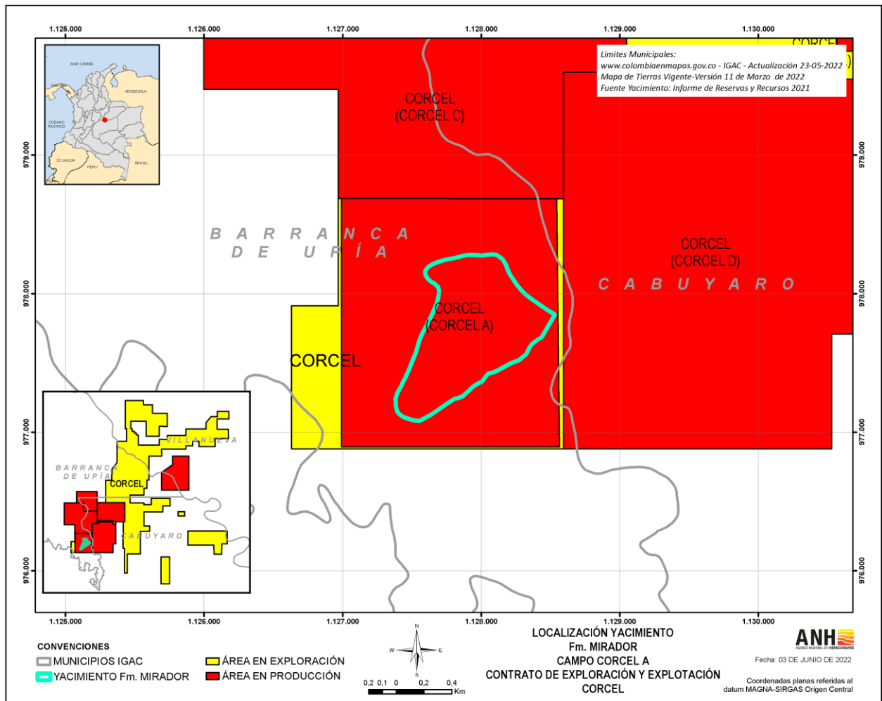
Figura. Localización Yacimiento Fm Mirador – Campo Corcel A
