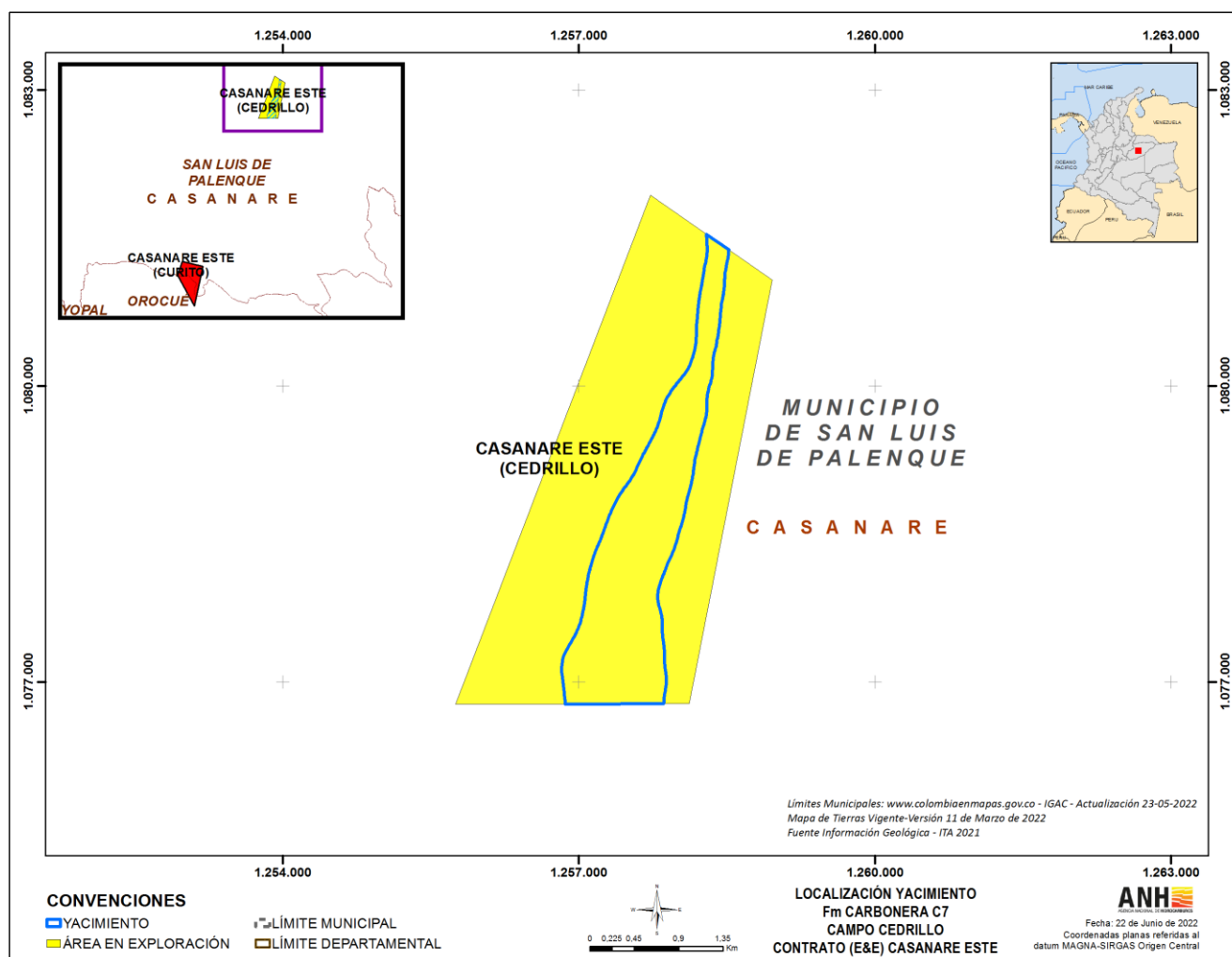
Figura. Localización Yacimiento C7 de la Fm. Carbonera – Campo Cedrillo
