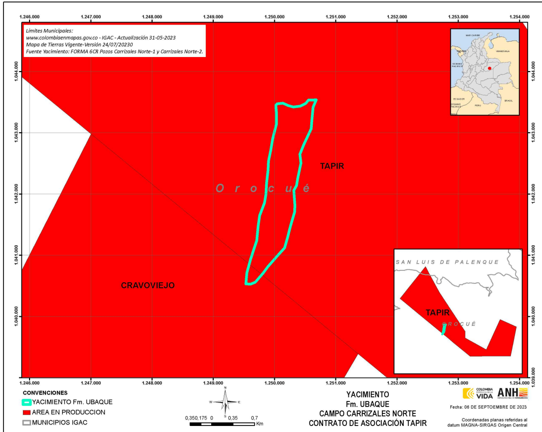
Figura 2. Localización Yacimiento Formación Ubaque – Campo Carrizales Norte
