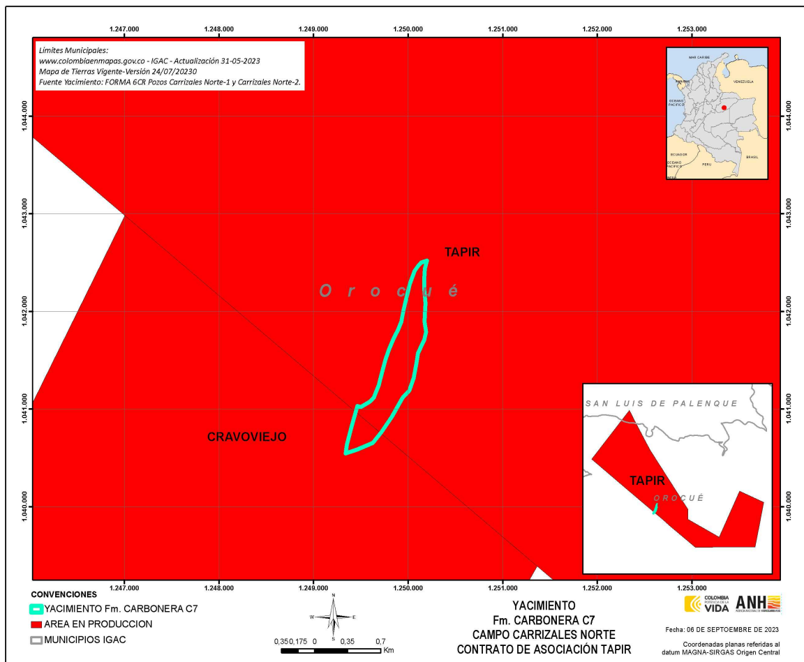
Figura 1. Localización Yacimiento C7 Formación Carbonera – Campo Carrizales Norte
