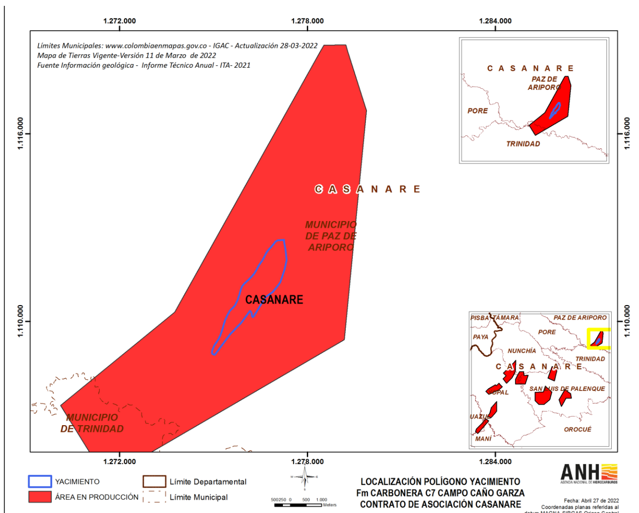
Figura 2. Localización Polígono Yacimiento Fm. Carbonera C7 – Campo Caño Garza, Contrato de Asociación Casanare.
