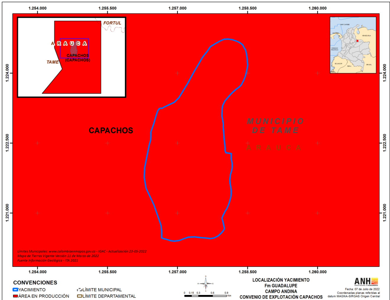
Figura. Localización Yacimiento Guadalupe, Fm Guadalupe – Campo Andina
